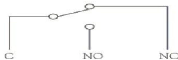
电路简图
