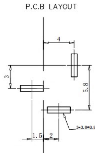
按点示意图 SCHEMATIC
