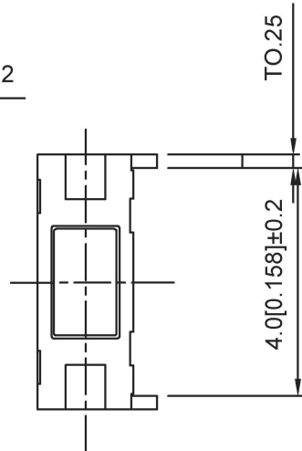
P.C.B LAYOUT
