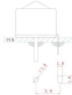
PCB焊锡插脚孔位
