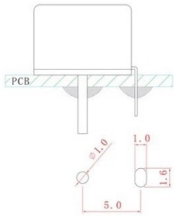
PCB焊锡插脚孔位
