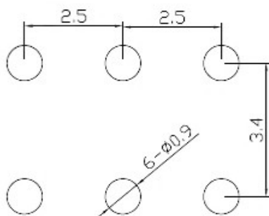
安装图 (PCB LAYOUT PLAN)
