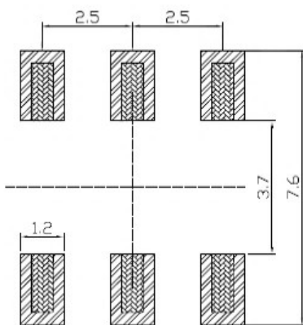
安装参考图
