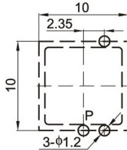
印制线路板
