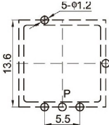
印制线路板 P.C.B
