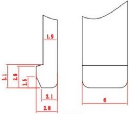
1.5: 1 锁舌参考规格
