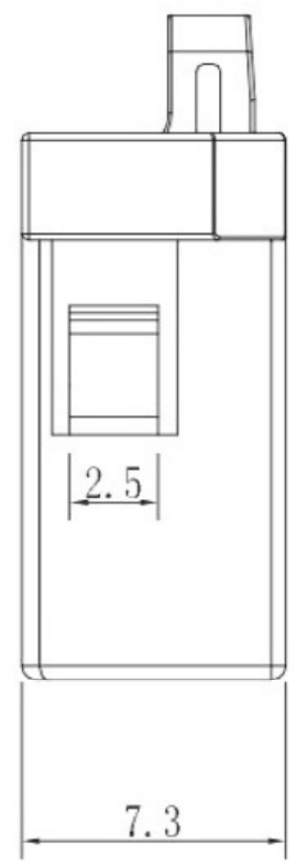
A-A 锁舌参考规格
