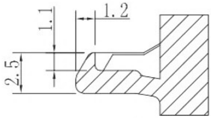
A-A 锁舌参考规格
