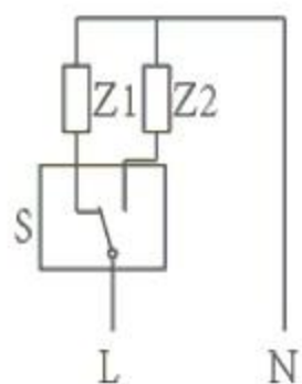
电路简图
