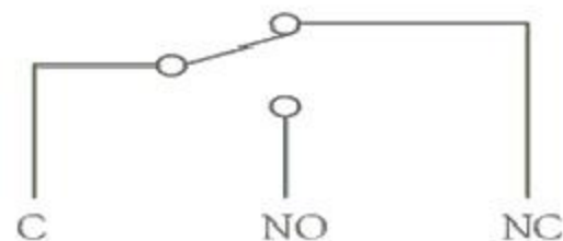
电路简图
