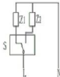
电路简图
