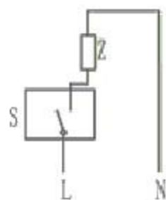
电路简图
