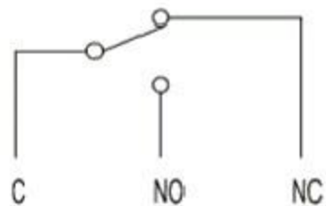
电路简图
