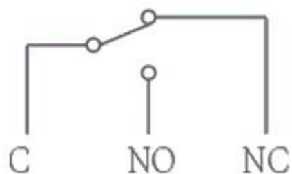
电路简图
