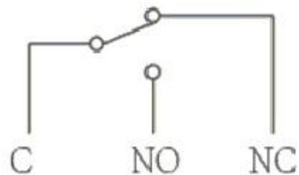
电路简图
