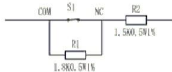
电路简图
