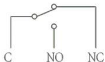
电路简图
