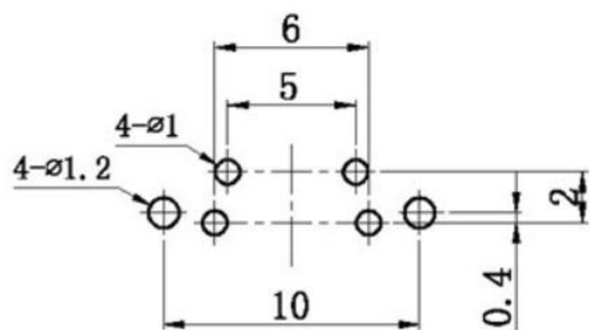
※ PCB板安装孔图
