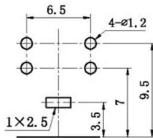
PCB板安装孔图
