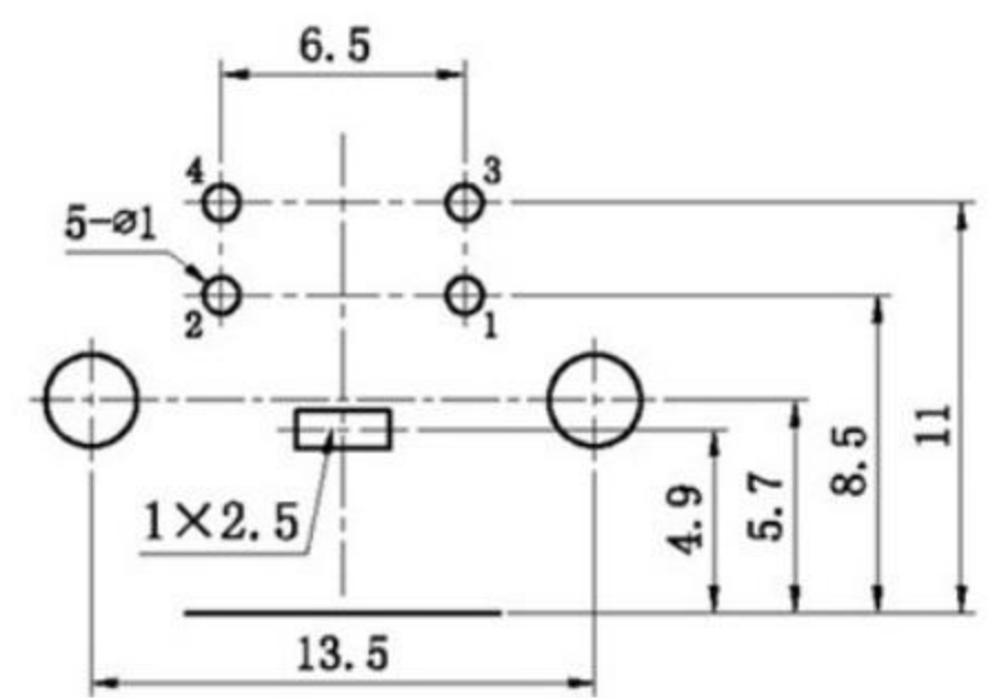
PCB板安装孔图
