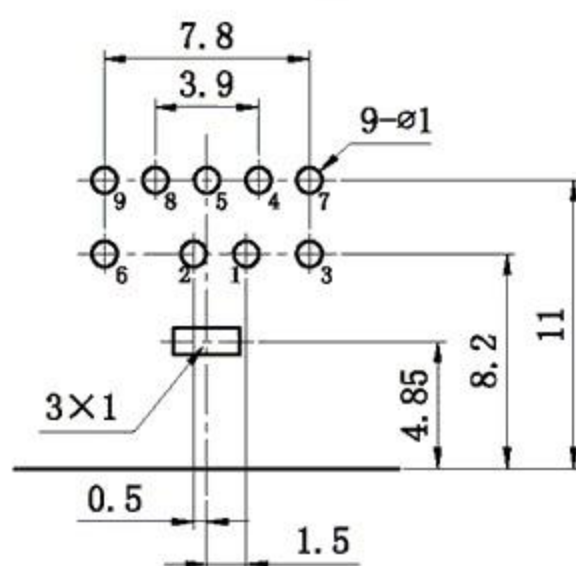
PCB板安装孔图
