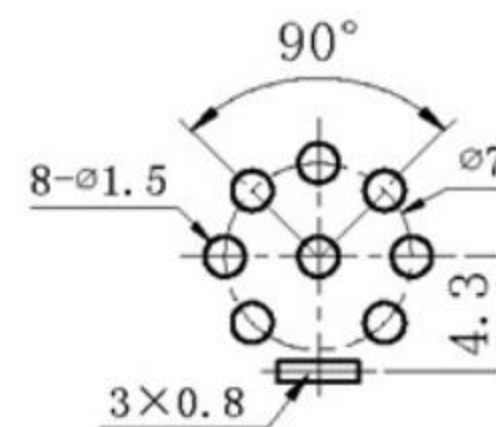
PCB板安装孔图
