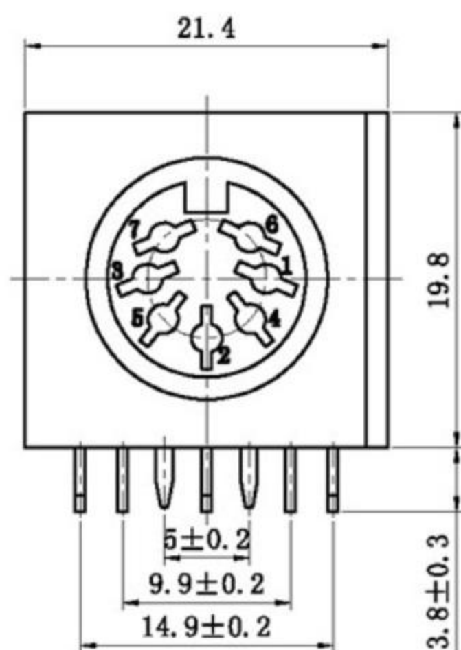
PCB板安装孔图
