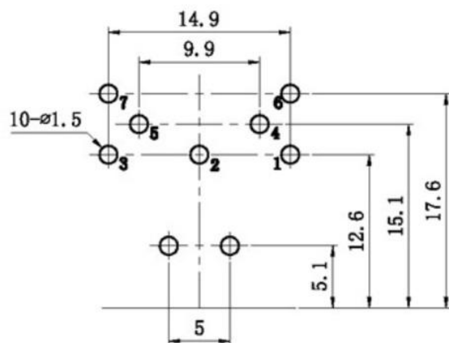
PCB板安装孔图
