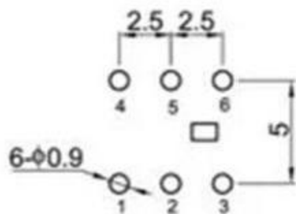
印制电路板 printed-circuit board
