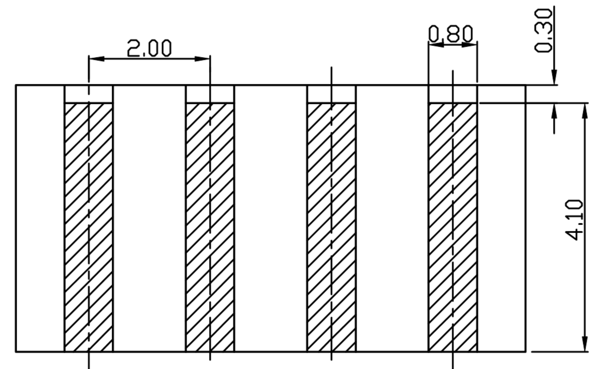
图为焊盘位置和大小
