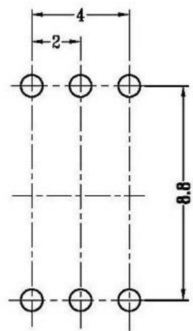
P.C.B LAYOUT TOP VIEW 注：“*”表示关键尺寸(3个).
