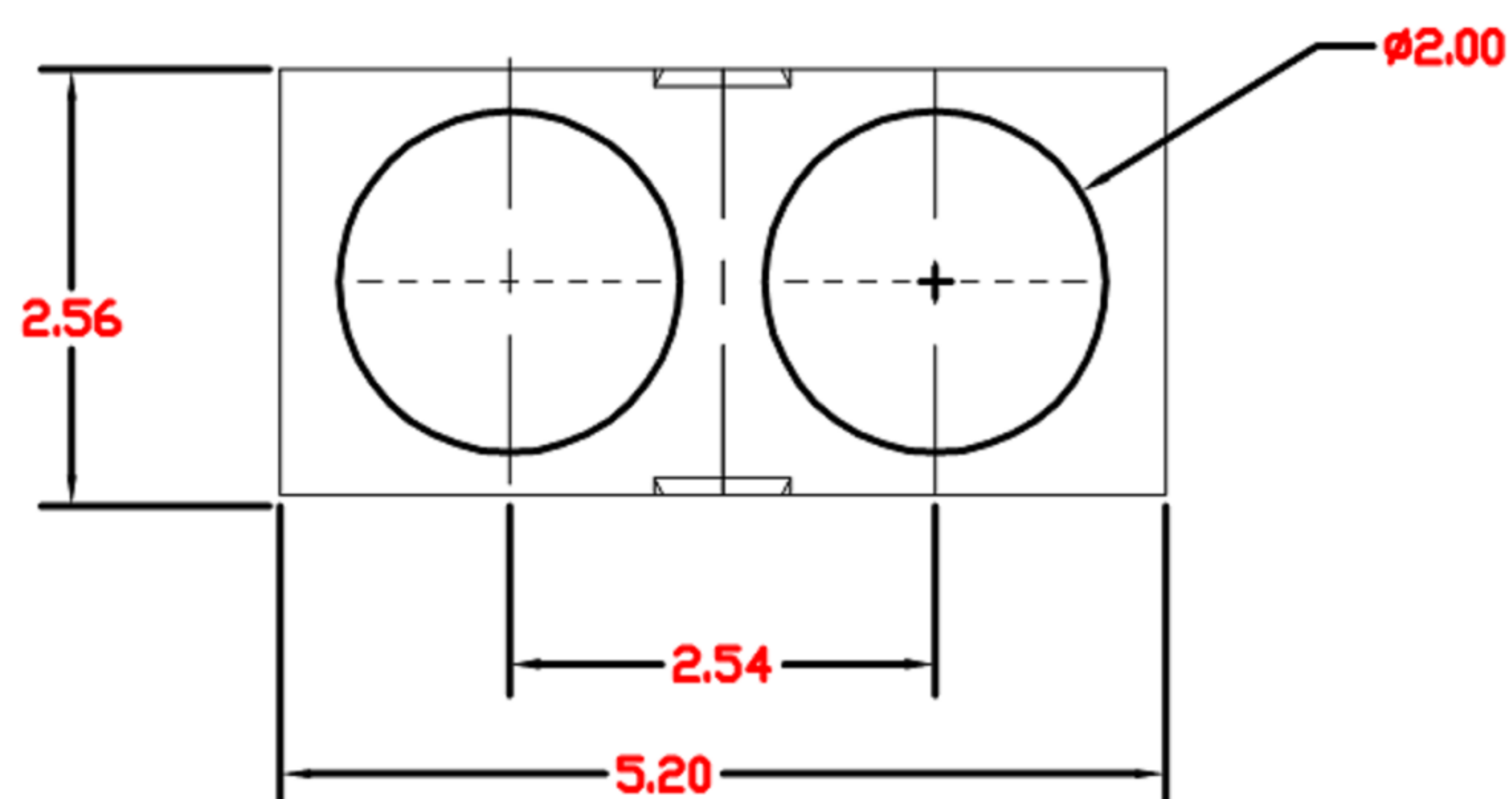
P.C.B.LAYOUT
