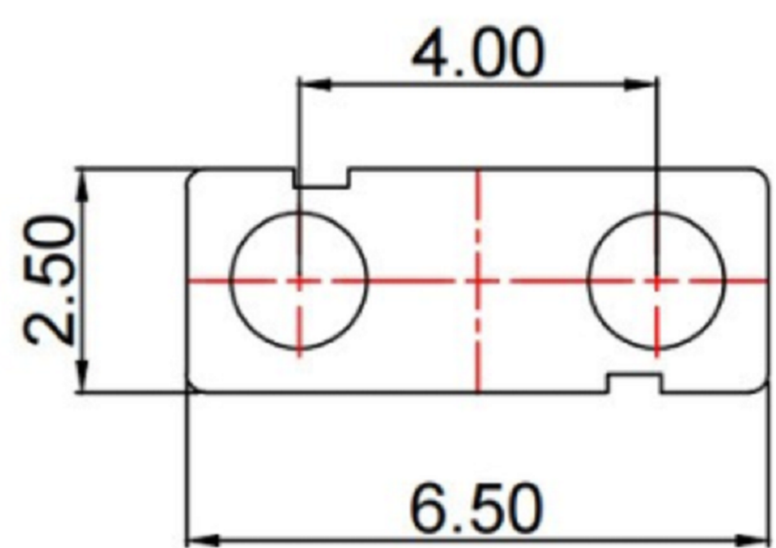
图为焊盘位置和大小
