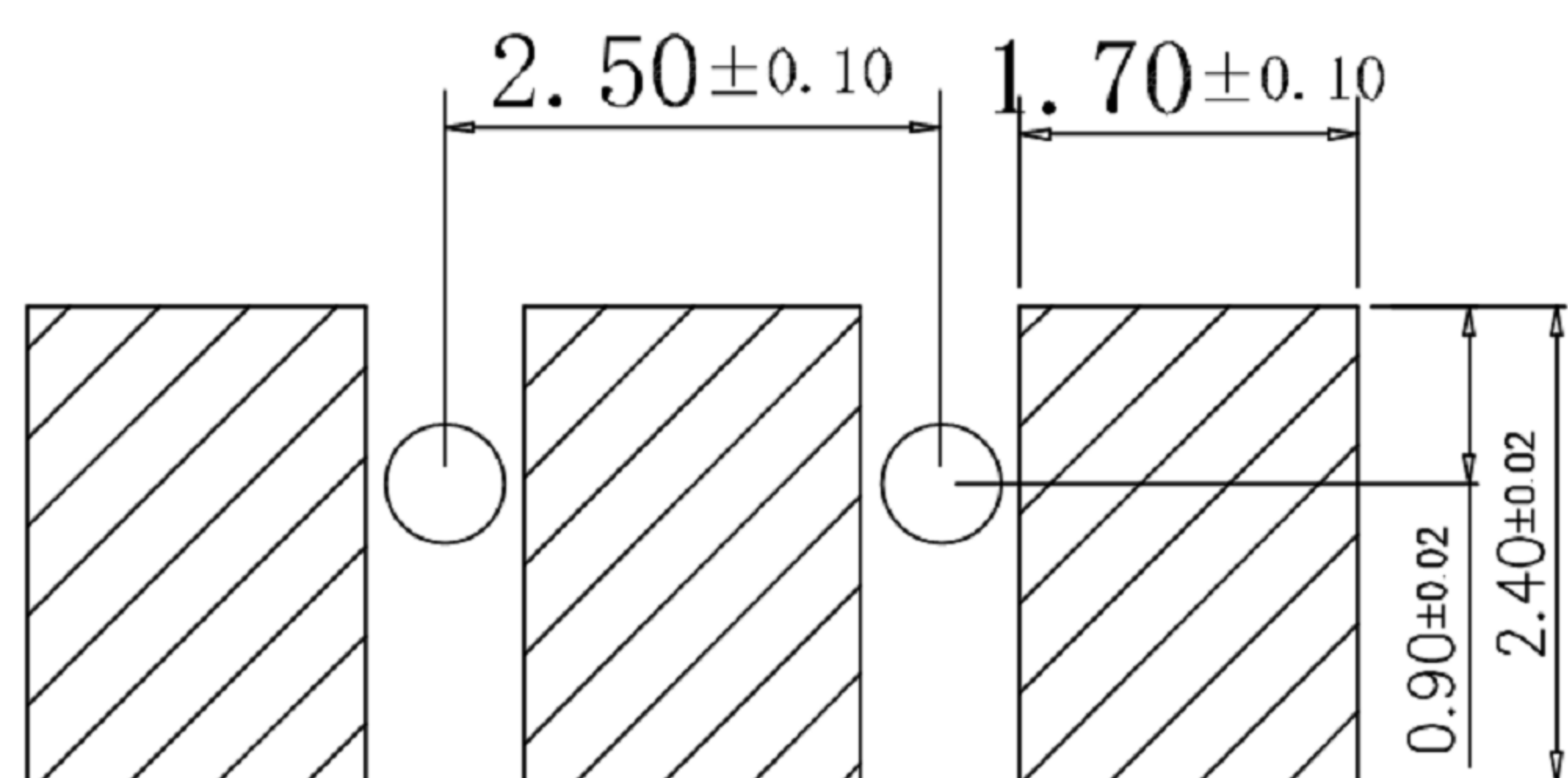
图为焊盘位置和大小
