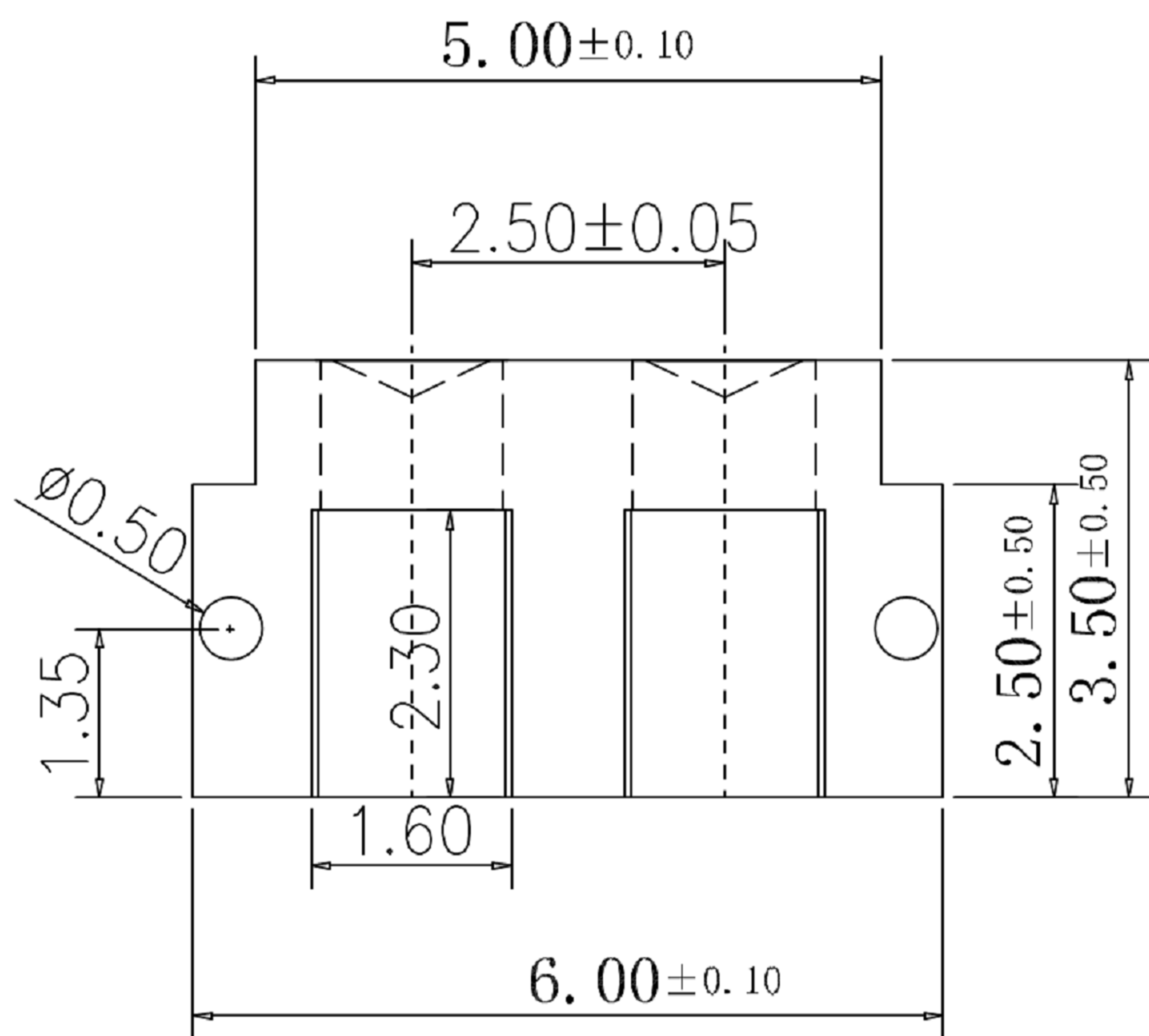
图为焊盘位置和大小
