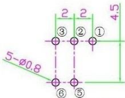
P.C.B 设计参考尺寸
