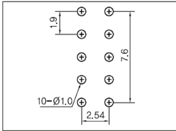
P.C.B DIMENSION
