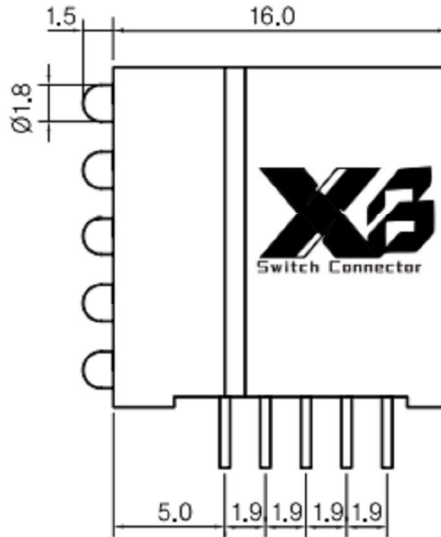
P.C.B DIMENSION
